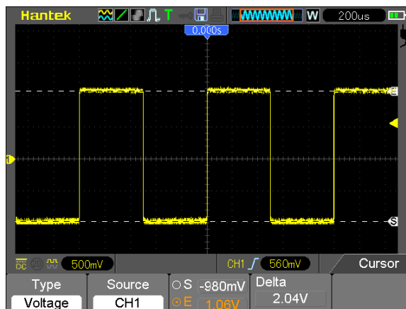
Курсор Voltage
